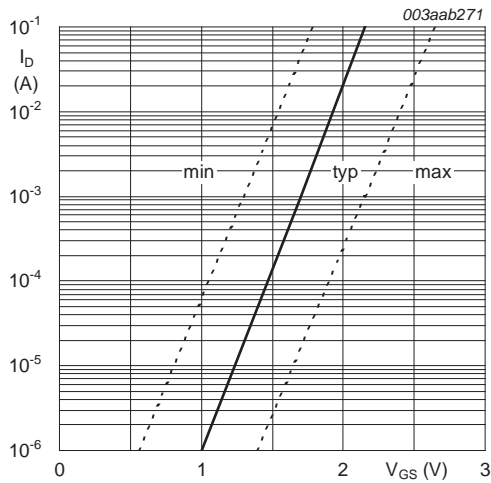
T_j = 25\text{ }^\circ\text{C}; V_{DS} = 5\text{ V}
