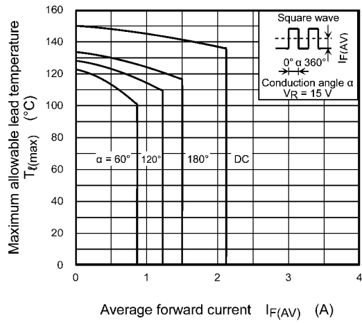
Fig. 10.4 T_{l(max)} - I_{F(AV)}
